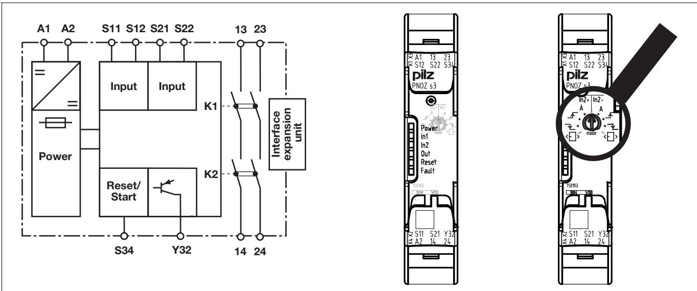
Mitte: Frontansicht mit Abdeckung Rechts: Frontansicht ohne Abdeckung
