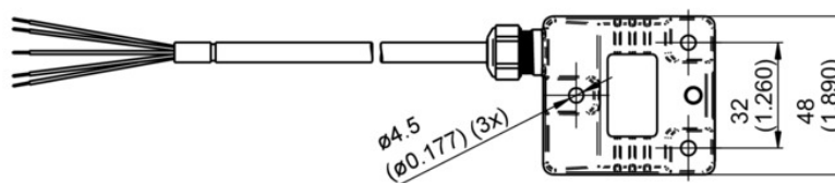
GIM500R - cable
